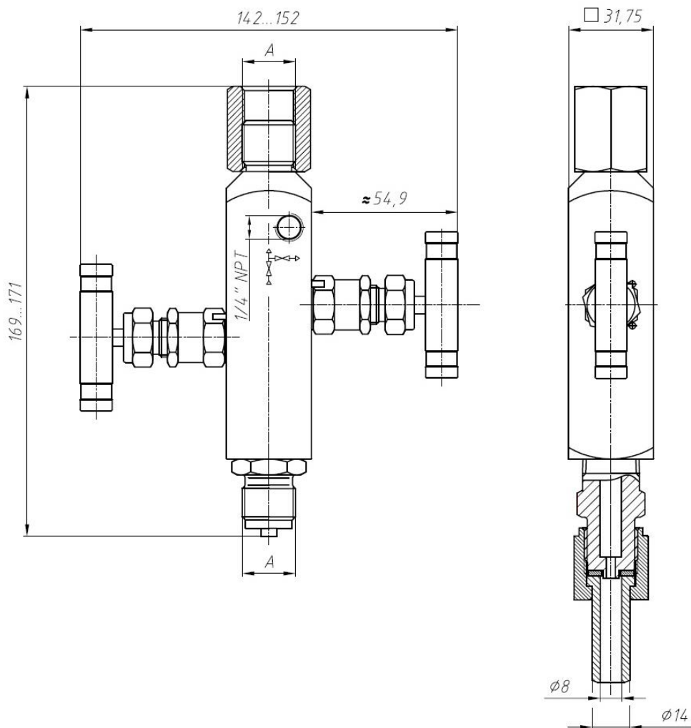
2-вентильный блок (присоединительные размеры: A – M20x1,5; G1/2")
