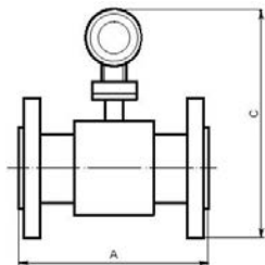
Рисунок Б.1 – Габаритные размеры фланцевого исполнения
