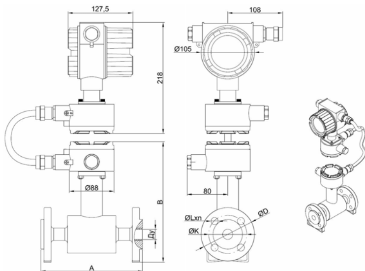
Рисунок Б.15 – Габаритные размеры взрывозащищенного расходомера (корпус 2)
