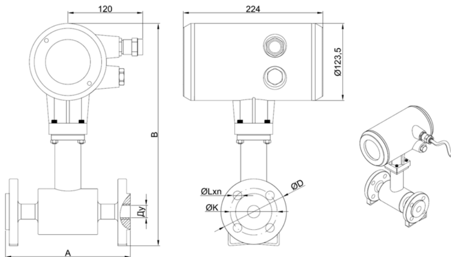
Рисунок Б.12 – Габаритные размеры взрывозащищенного расходомера (корпус 1)
