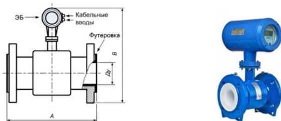
Рисунок Б.2 – Вид конструкции сенсора с установленным стандартным ЭБ
