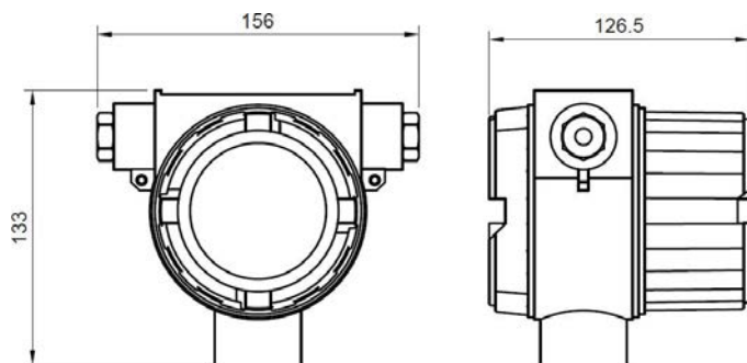
Рисунок Б.9 – Внешний вид и габаритные размеры корпуса электронного блока
