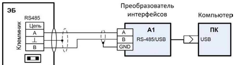
Рисунок Г.10 – Схема подключения расходомера к ПК
