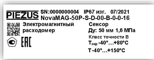
Рисунок 10.1 – Примеры идентификационных наклеек на корпусах для отдельного исполнения компонентов расходомера: а) на электронный блок; б) на датчик сенсора
