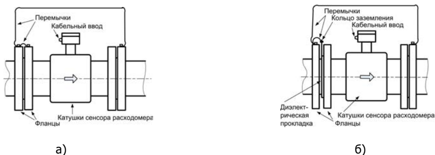
Рисунок 5.10 – Схема соединения фланцев при использовании катодной защиты (элементы крепежа на фланцах не показаны): а) без металлических колец; б) с одним электропроводным кольцом и диэлектрическими прокладками
