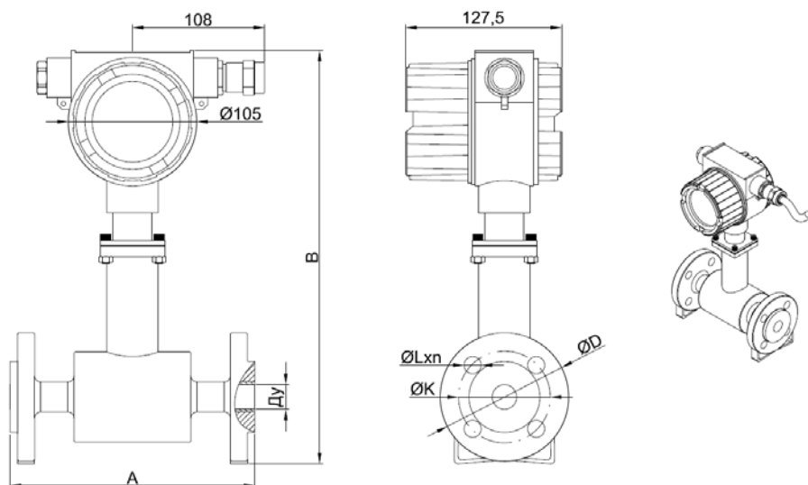
Рисунок Б.13 – Габаритные размеры взрывозащищенного расходомера (корпус 2)
