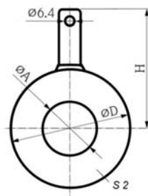
Рисунок Б.11 – Габаритные размеры заземляющих дисков (колец) для фланцевых соединений с Ду от 700 мм (A, D, H – размеры для справок)
