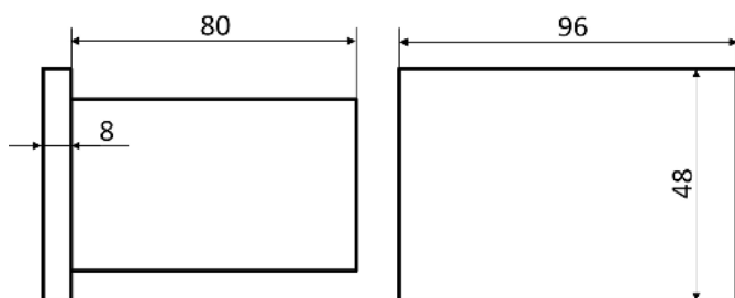
Габаритные размеры корпуса
