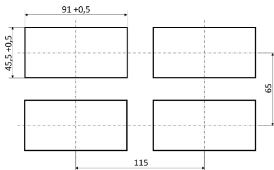
Разметка окон в щите для установки индикаторов
