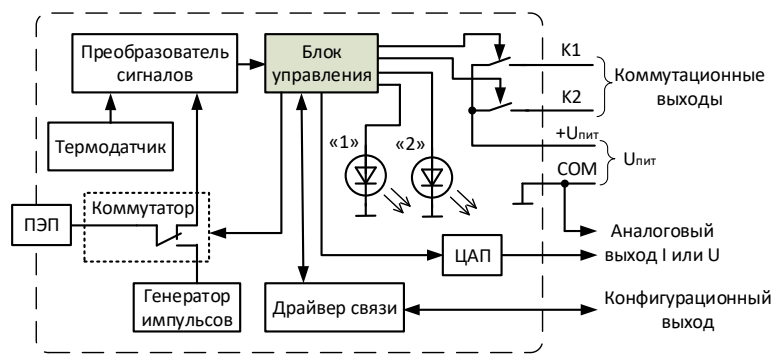
Рисунок 2 – Структурная схема датчика
