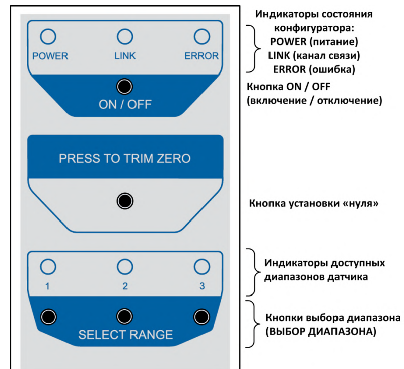
Рисунок А.2 – Назначение элементов управления лицевой панели
