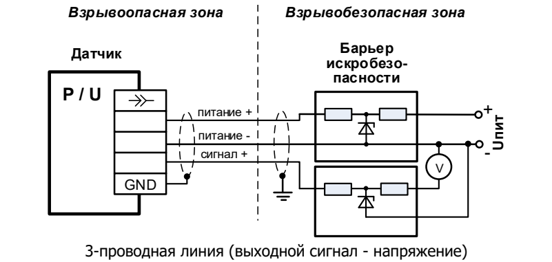
Рисунок А.2 – Пример схемы подключения аналогового выхода сигнала «напряжение»
