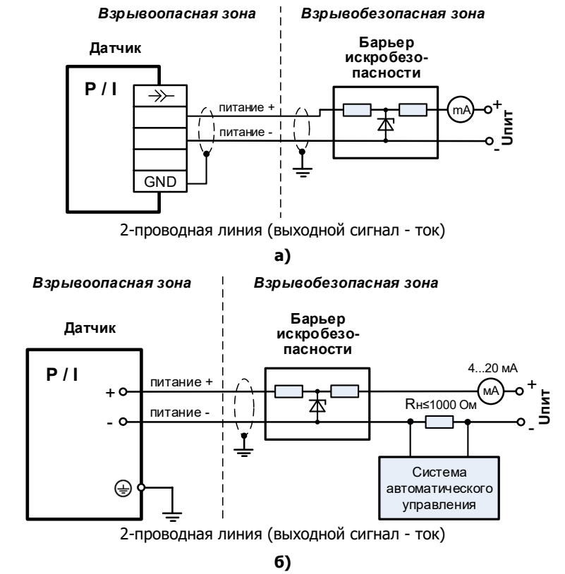
Рисунок А.1 – Примеры схем подключения аналоговых выходов сигнала «ток»: а) для разъема DIN 43650А; б) для кабельного ввода
