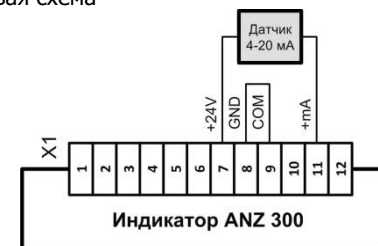
Рисунок Б.1 – Подключение прибора
