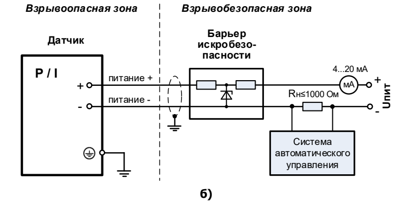
Рисунок А.1 – Примеры схем подключения аналоговых выходов сигнала «ток»: а) для разъема DIN 43650А; б) для кабельного ввода
