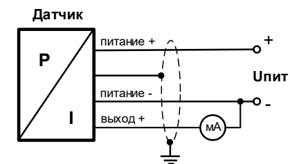
3-проводная линия (выходной сигнал – ток)
