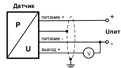
3-проводная линия (выходной сигнал – напряжение)
