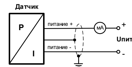
2-проводная линия (выходной сигнал – ток)
