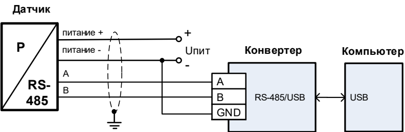
Рисунок 2 – 4-проводная линия (выходной сигнал – RS-485)
