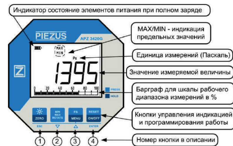
Рисунок 1 – Назначение элементов лицевой панели прибора
