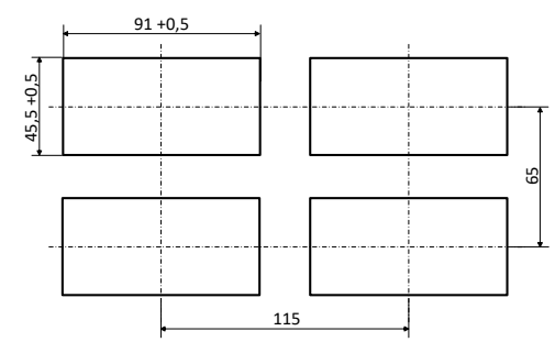
Габаритные размеры корпуса.
