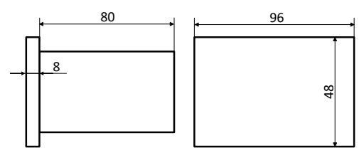
Габаритные размеры корпуса.
