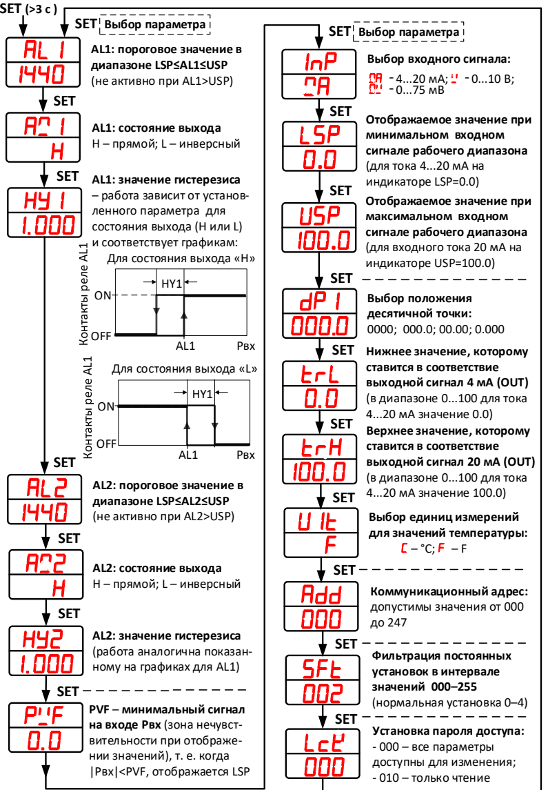
Рисунок 3 – Структура меню настройки прибора (*демпфирование – время установления выходных значений (показаний) при ступенчатом изменении сигнала на входе – P вх )
